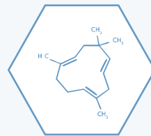
Humulene
