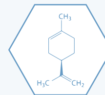
Limonene
