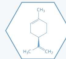
Limonene
