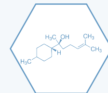
a-Bisabolol
