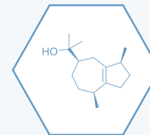
(-)-Guaiool
