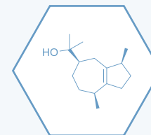
(-)-Guaiol
